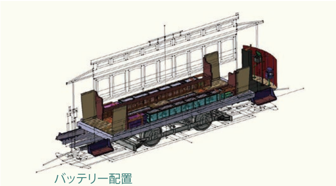
バッテリー配置 Battery layout
