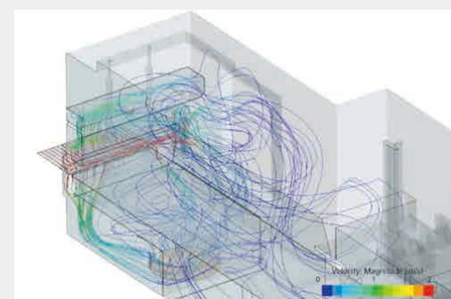
内部気流 CFD解析 Internal Airflow CFD Analysis
